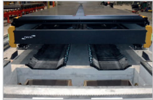
Chip automatic extraction Extracción automática de viruta
