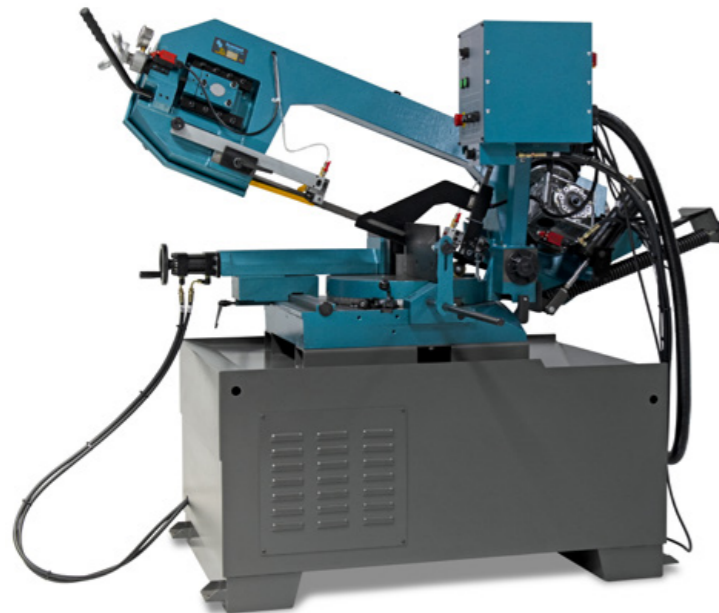
SCANTOOL 420 GSHT Semi Auto with "One Touch" auto operation Båndsave til metal med hydraulisk skruestik, 0 - 60° Band saws for metal with Hydraulic vise, 0 - 60° Bandsäge für Metall mit manuellem Schraubstock, 0 - 60°
